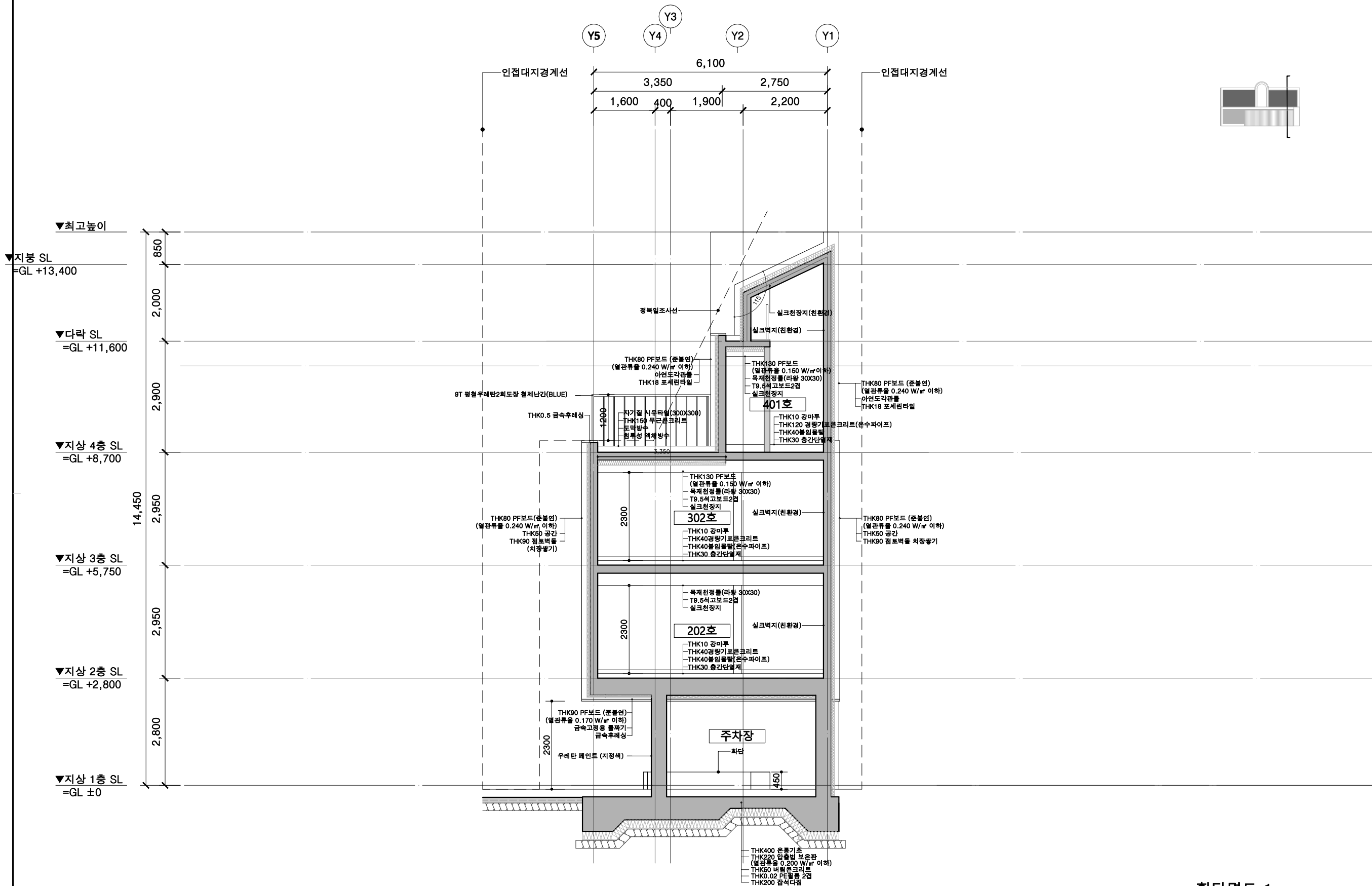
횡단면도-1 1/100
